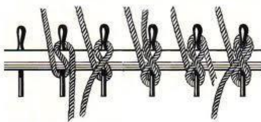
Rys. 18. Poprawne knagowanie
