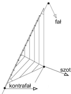
Rys. 15. Olinowanie ruchome - sztaksle dziobowe
