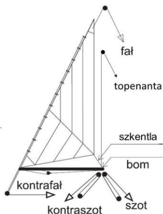
Rys. 16. Olinowanie ruchome - sztaksle na bomach
