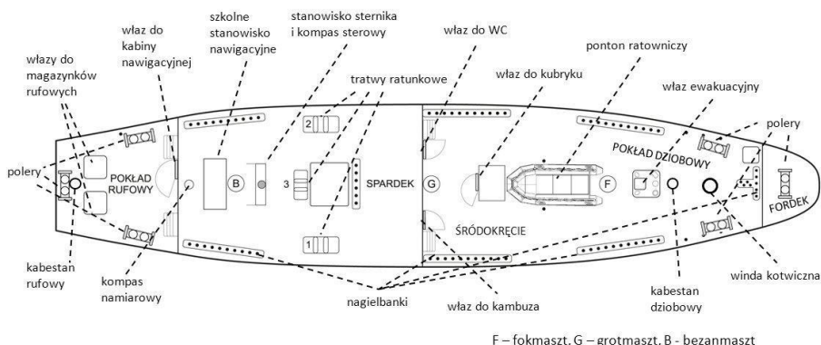
Rys. 8 Pokład i urządzenia pokładowe
